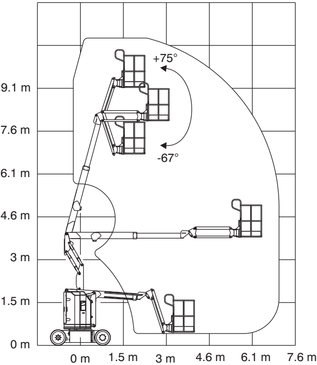
旋转短臂运动范围
