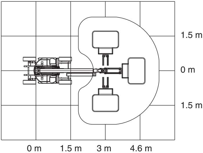
旋转短臂运动范围
